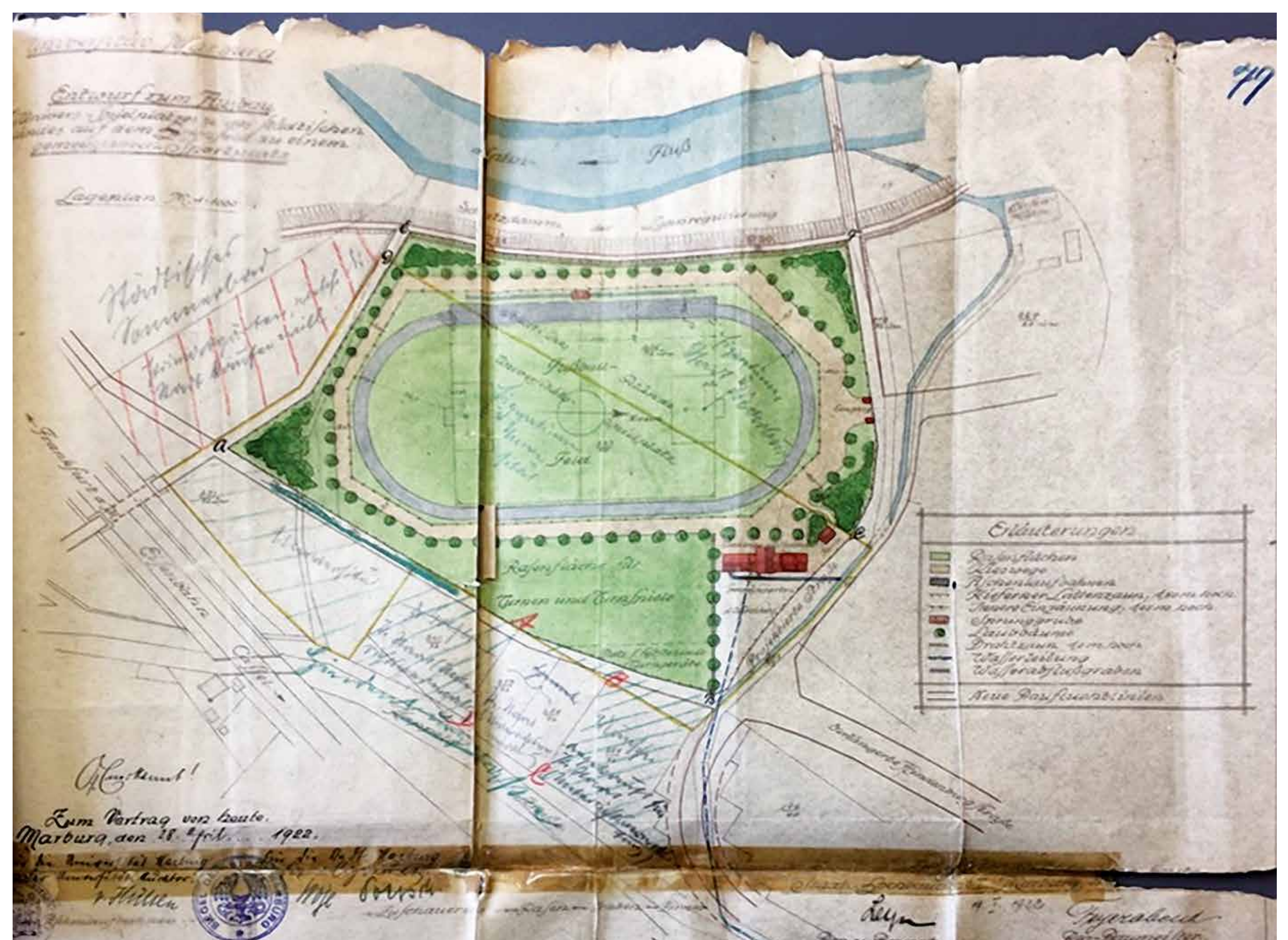
Der gemeinsame Plan (1922) umfasste schon den Flächenanteil von Universität und Stadt, sah auch ein Umkleidegebäude und eine umfassende Grünflächengestaltung vor. Die eingezeichnete Diagonale kennzeichnet die jeweiligen Anteile.
